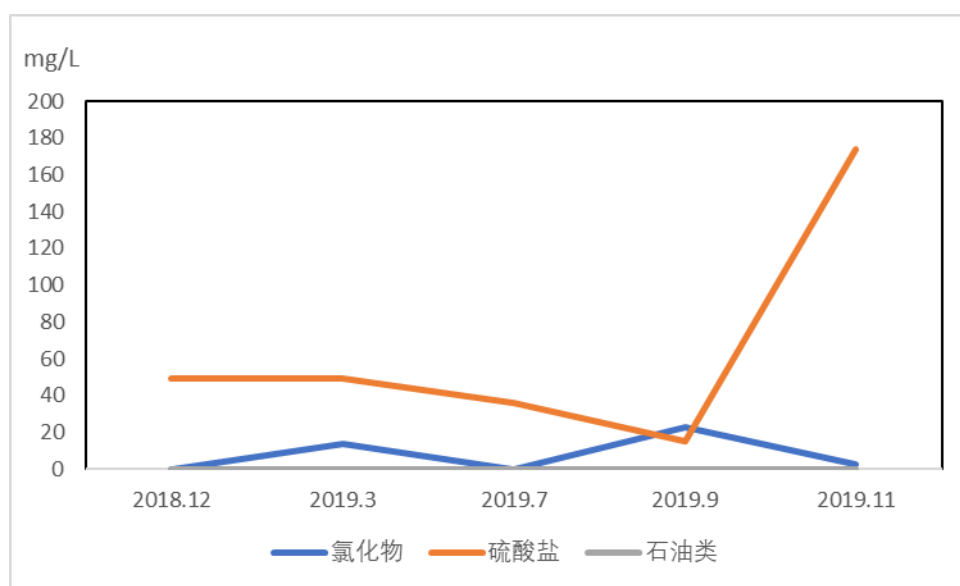
图 8-4 硫酸盐、氯化物、石油类变化趋势图
