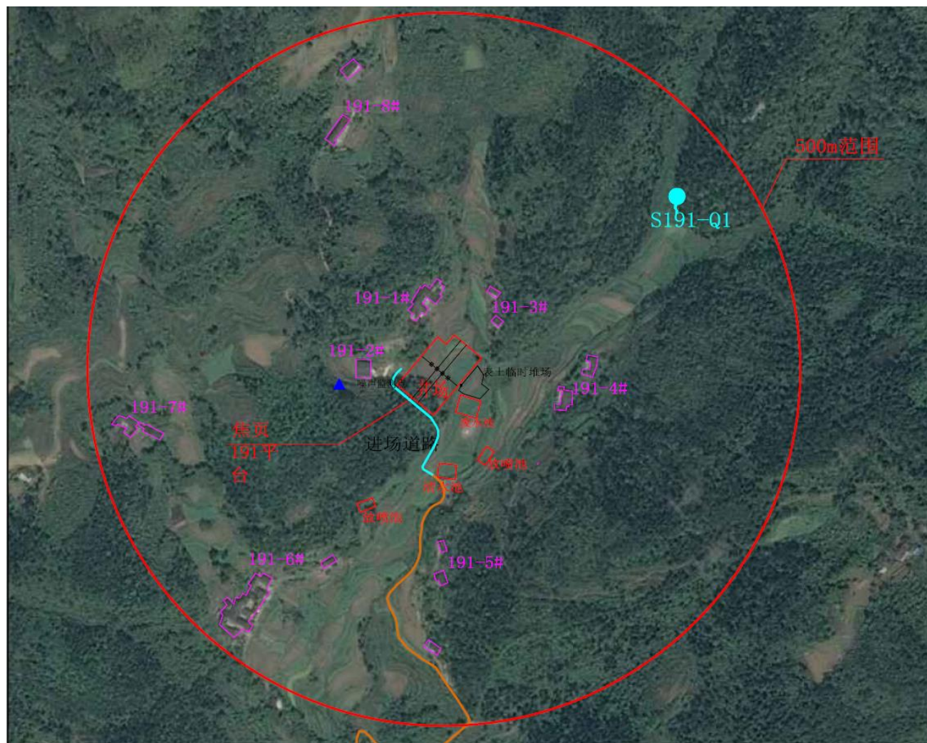
图 1.8-3 焦页 191#平台敏感点分布示意图
