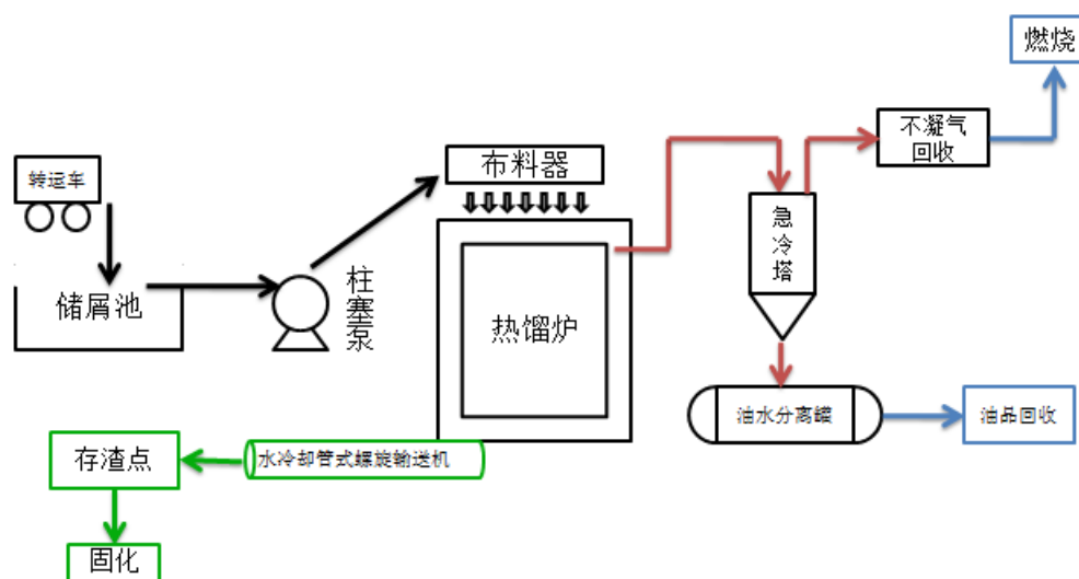
图 9.1-1 油基钻屑处理工艺流程图
