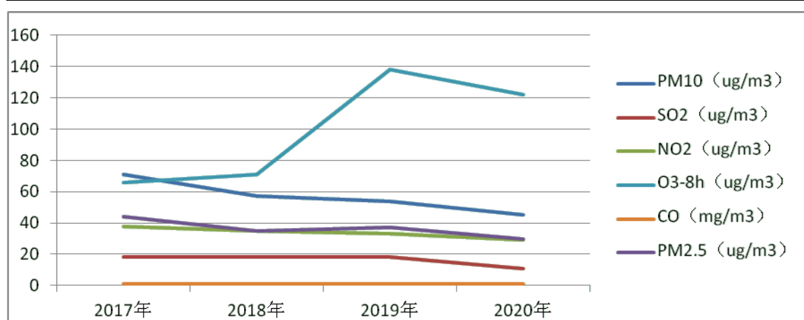
图 8-1 2017 年至 2020 年涪陵区环境空气污染物年际变化
