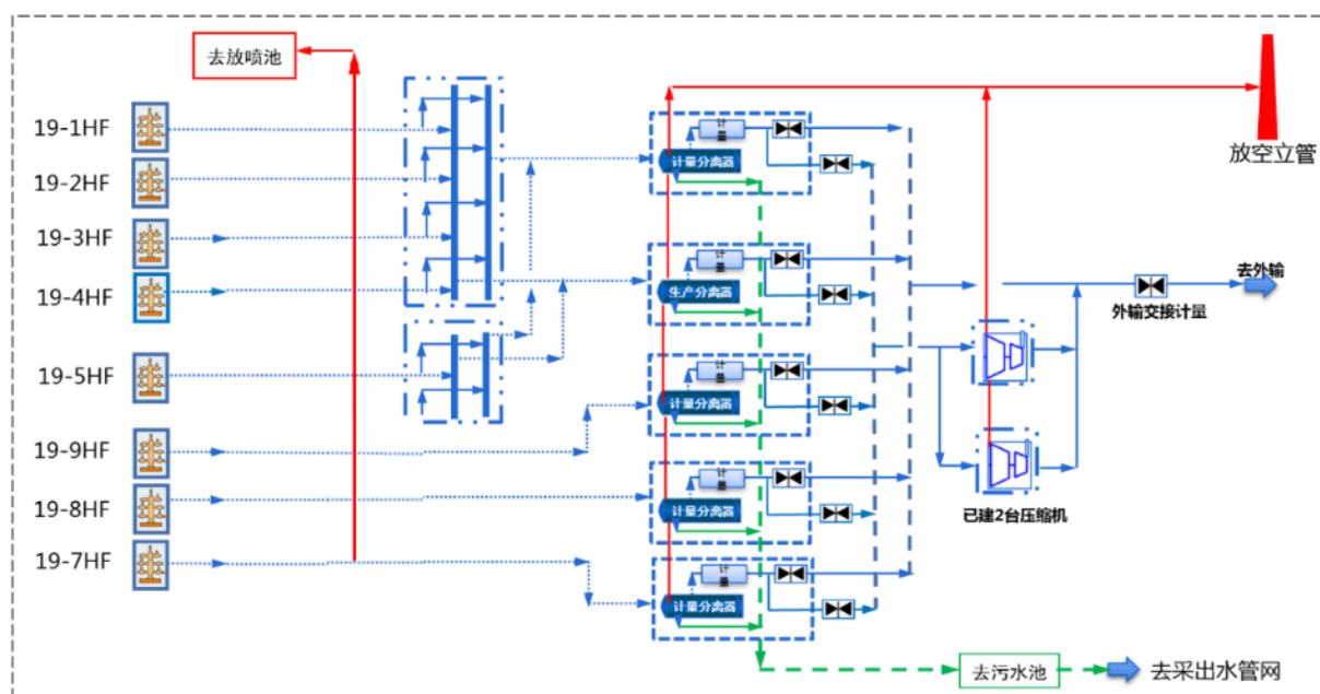
图 2.1-3 焦页 19 号集气站工艺流程图
