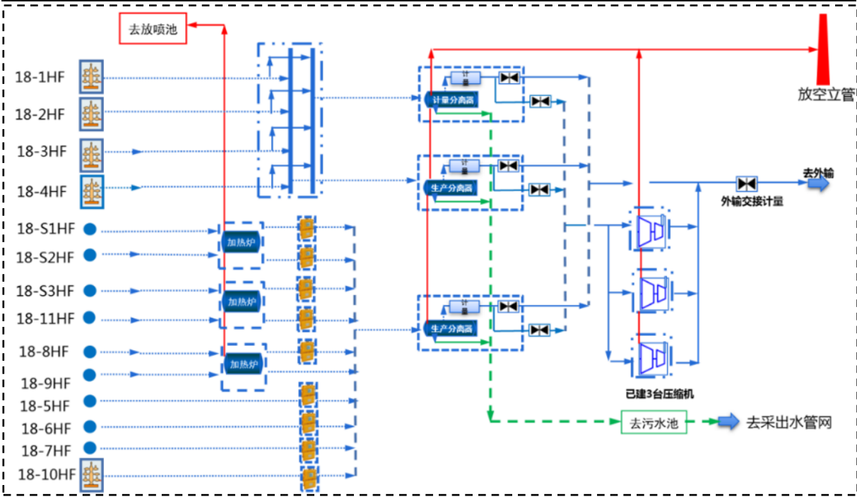
图 2.1-1 焦页 18 号集气站工艺流程图
