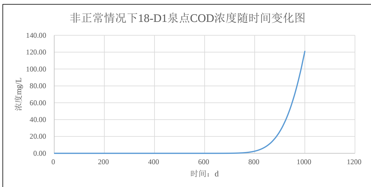
图 4.2-1 非正常情况下 18-D1 泉点 COD 浓度随时间变化图
