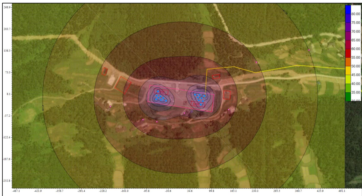
图 4.4-4 焦页 19 号扩井组柴油发电机钻井时各场界噪声模拟预测图
