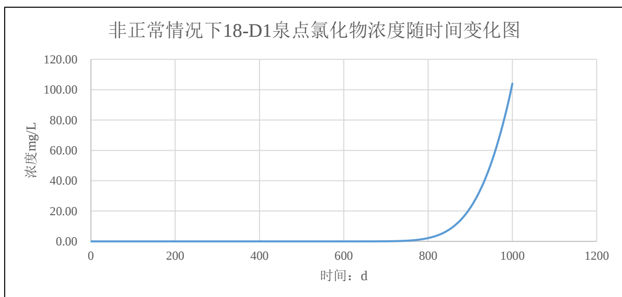
图 4.2-2 非正常情况下 18-D1 泉点氯化物浓度随时间变化图
