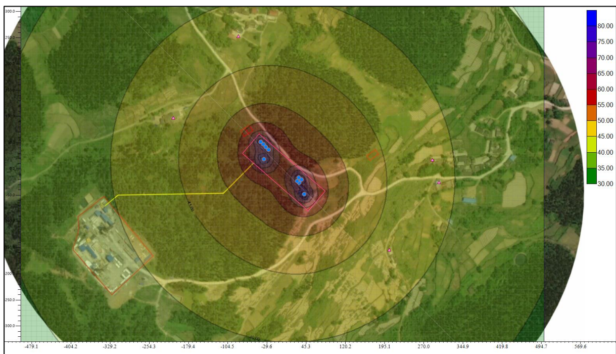
图 4.4-1 焦页 18 号东井组网电钻井时各场界噪声模拟预测图
