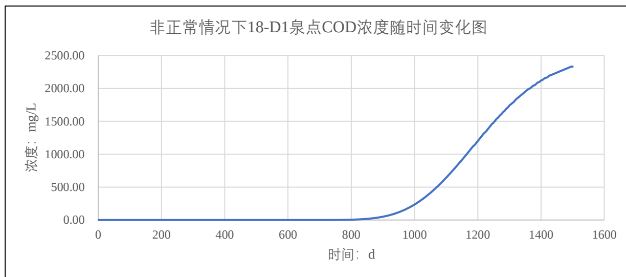
图 4.2-3 非正常情况下 18-D1 泉点 COD 浓度随时间变化图
