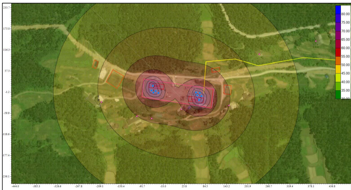
图 4.4-3 焦页 19 号扩井组网电钻井时各场界噪声模拟预测图
