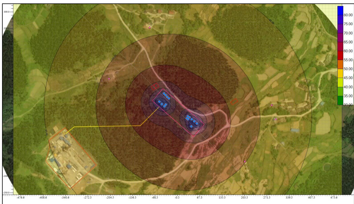
图 4.4-2 焦页 18 号东井组柴油发电机钻井时各场界噪声模拟预测图
