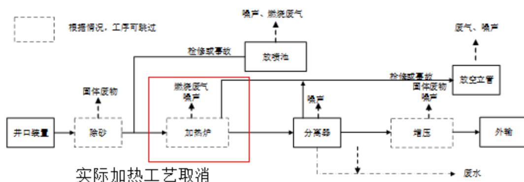
图 2.6-1 工艺流程图
